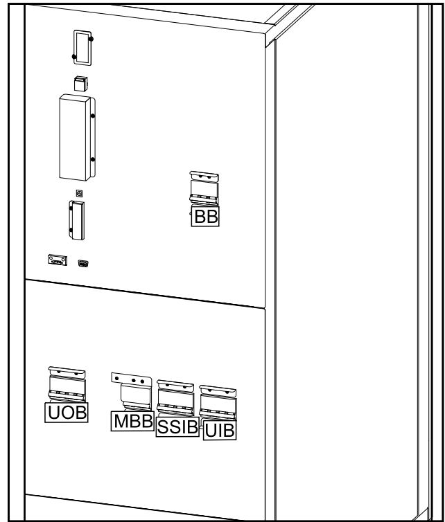
Vista posteriore dell'UPS da 20 kVA con batterie interne
