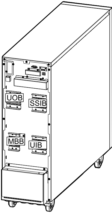
Vista posteriore dell'UPS da 20 kVA per batterie esterne
