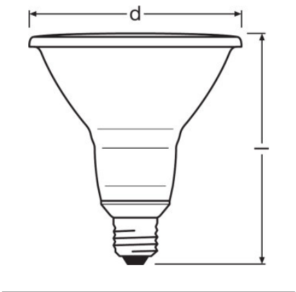
P PAR 38 100 15° 11 W/2700 K E27, P PAR 38 100 30° 12 W/2700 K E27
