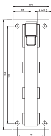
Vooraanzicht
