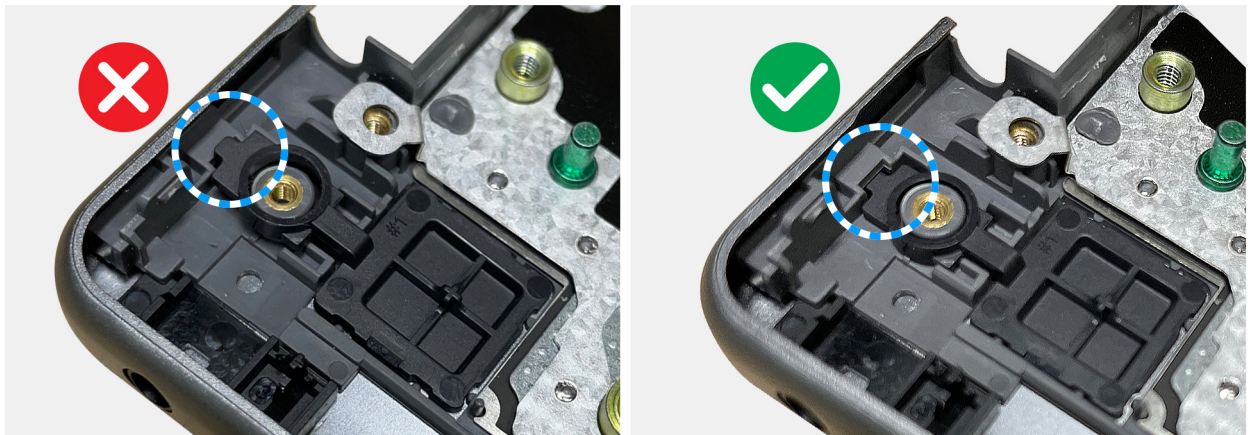
Figur 92. Installera strömbrytaren
