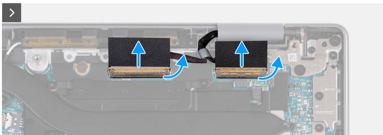
Figur 77. Ta bort bildskärmsenheten (för datorer som levereras med stöd för WWAN)
