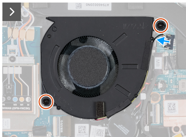
Figur 37. Ta bort fläkten (för datorer som levereras med stöd för WWAN)
