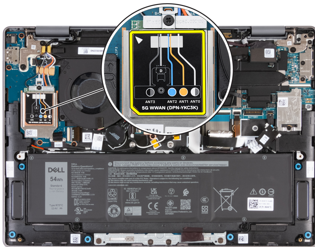
Figur 29. Antennkabelanslutningar
