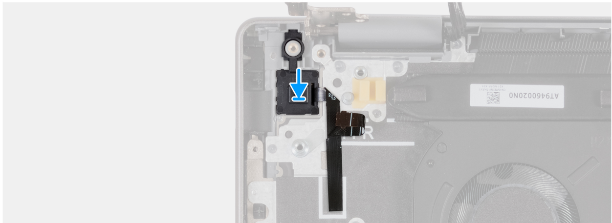
Figur 91. Installera strömbrytaren med fingeravtrycksläsare
