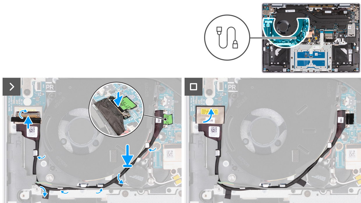
Figur 51. Installera I/O-kortkabeln (för datorer som levereras med stöd för endast WLAN)
