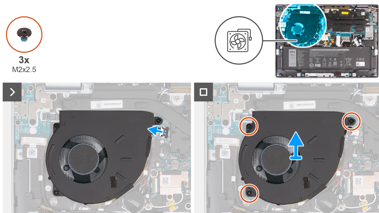
Figur 35. Ta bort fläkten (för datorer som levereras med stöd för endast WLAN)
