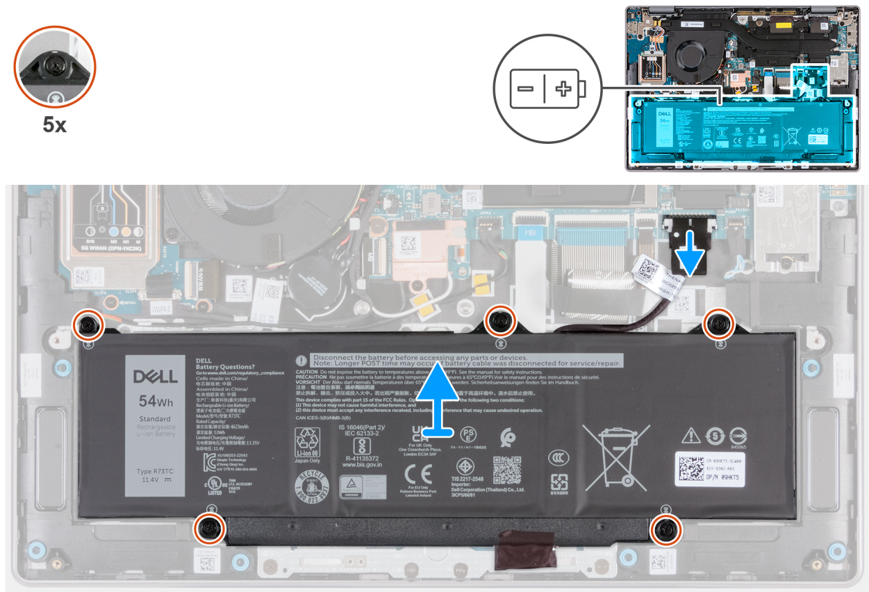
Figur 39. Ta bort batteriet
