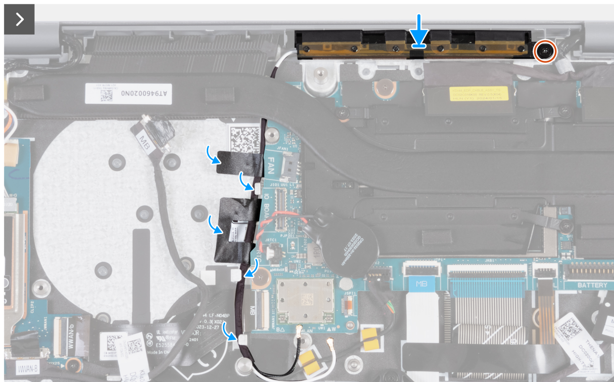
Figur 69. Installera WLAN-antenmodulen (för datorer som levereras med stöd för WWAN)
