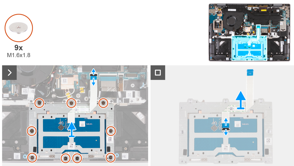
Figur 86. Ta bort styrplatteenheten
