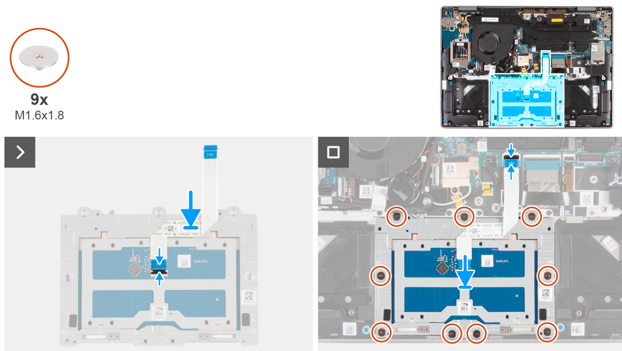
Figur 87. Installera styrplatteenheten
