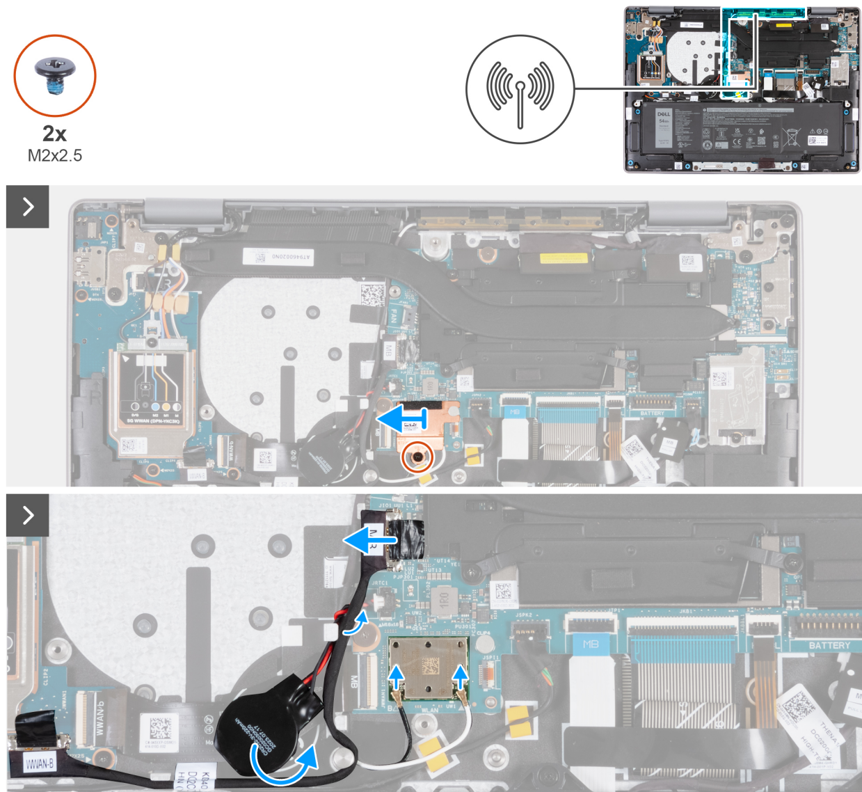
Figur 65. Ta bort WLAN-antenmodulen
