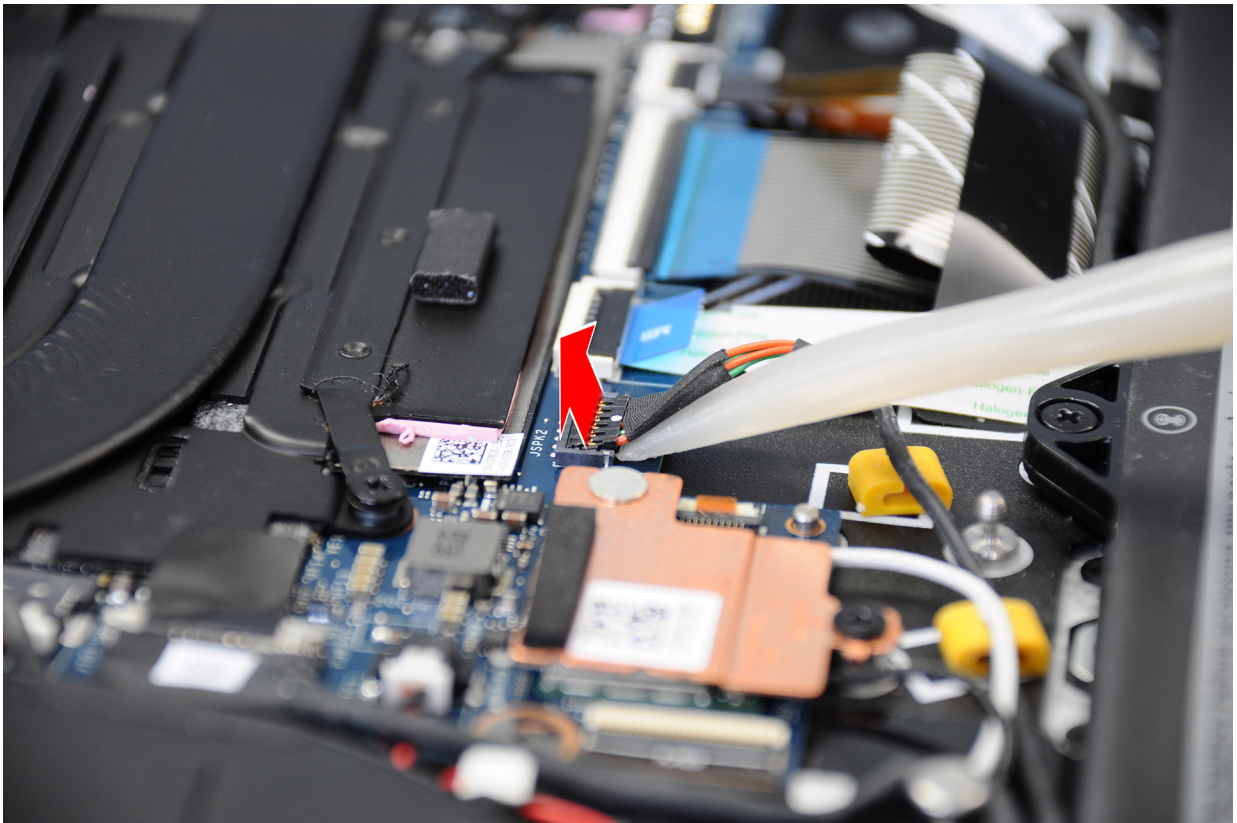
Figur 32. Bända bort högtalarkabeln från kontakten
