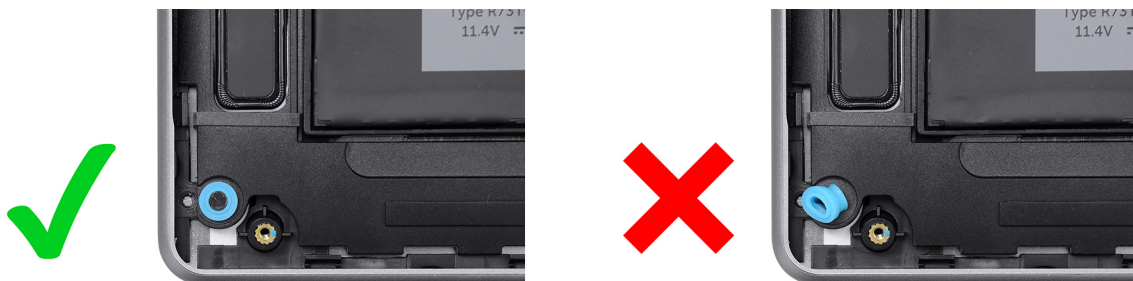
Figur 34. Installation av gummibussningar
