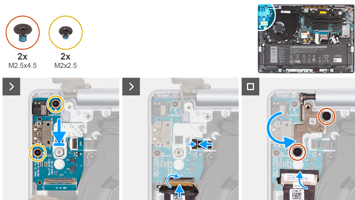
Figur 83. Installera I/O-kortet (för datorer som levereras med stöd för endast WLAN)
