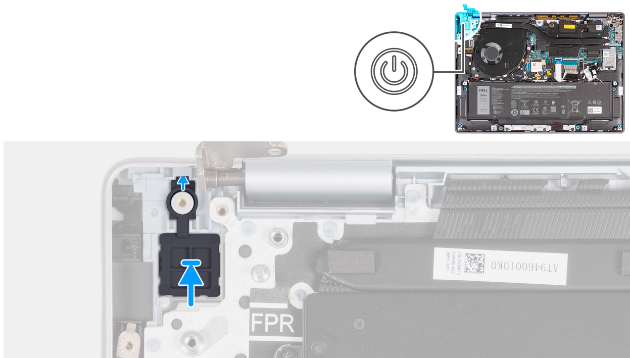
Figur 90. Installera strömbrytaren
