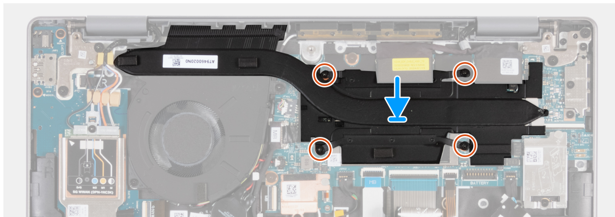
Figur 45. Installera kylflänsen
