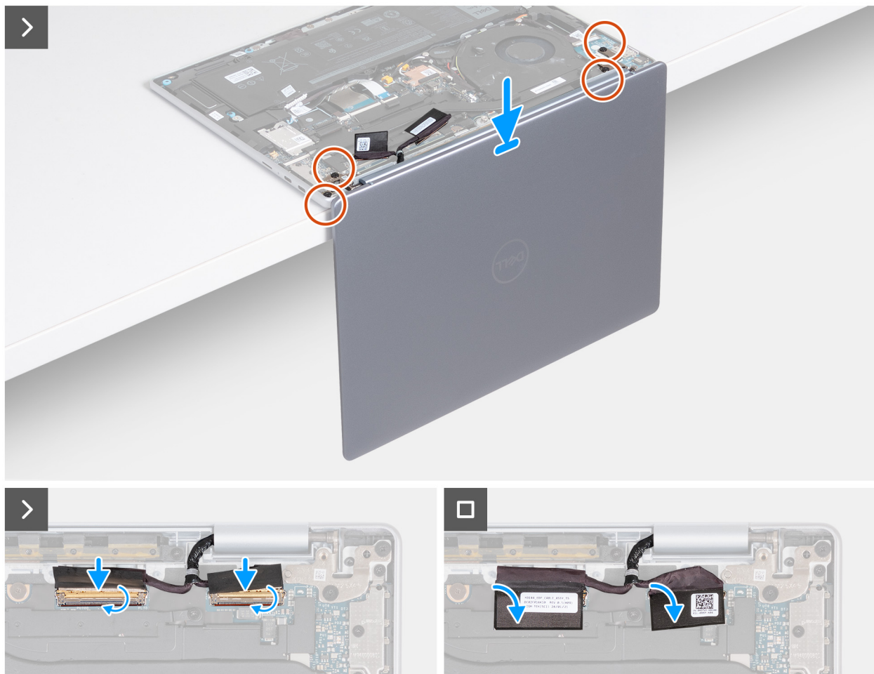
Figur 76. Installera bildskärmsenheten (för datorer som levereras med stöd för endast WLAN)
