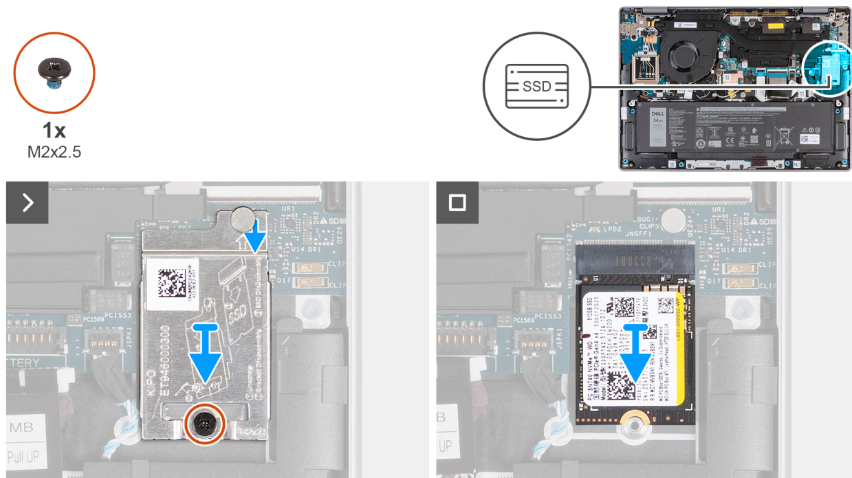
Figur 21. Ta bort SSD-disken
