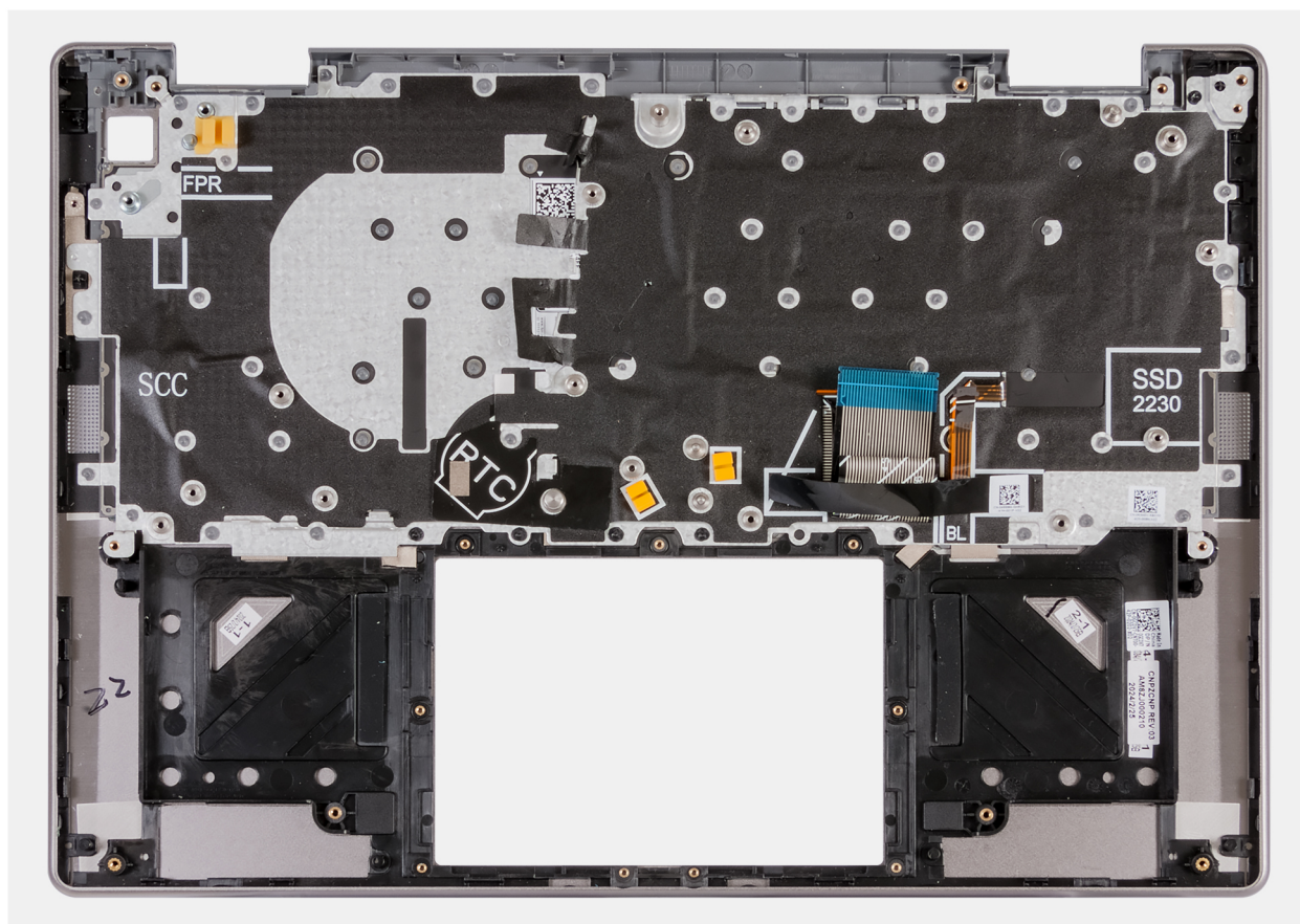
Figur 101. Handledsstöds- och tangentbordsenhet
