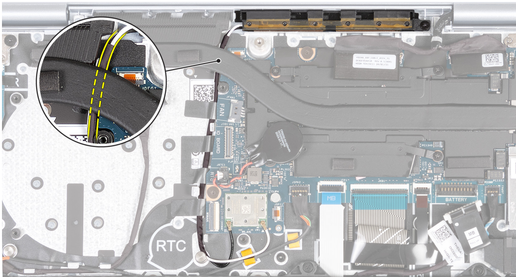
Figur 68. Ta bort WLAN-antennkablar
