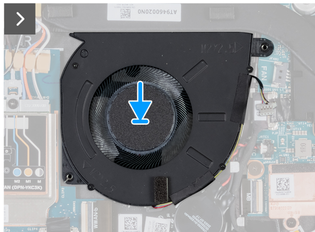
Figur 38. Installera fläkten (för datorer som levereras med stöd för WWAN)
