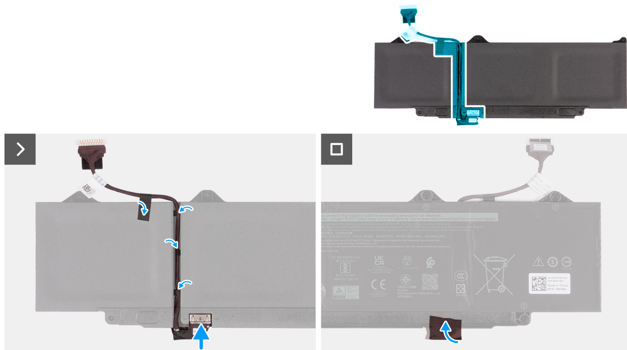
Figur 43. Installera batterikabeln
