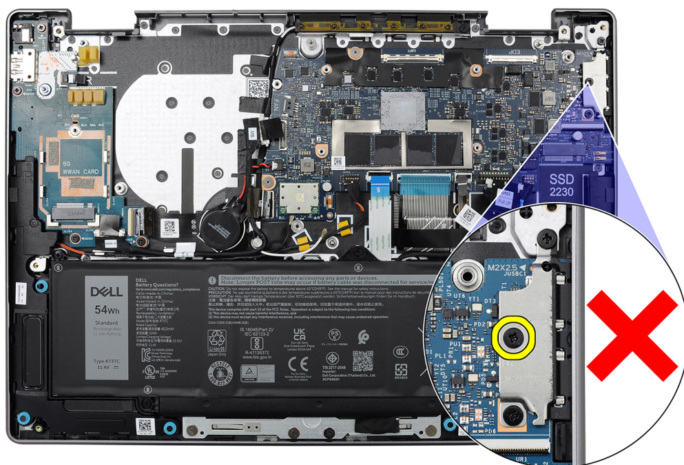
Figur 96. Fäste för USB Typ C
