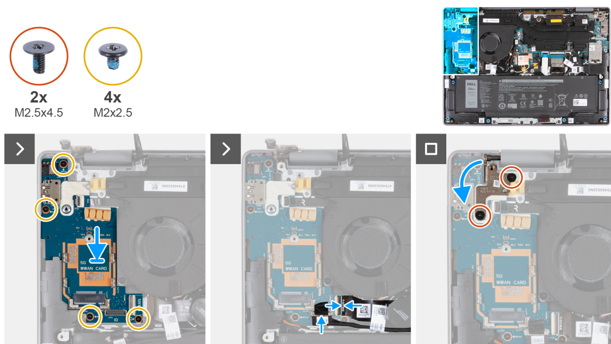
Figur 85. Installera I/O-kortet och ta bort I/O-kortet (för datorer som levereras med stöd för WWAN)
