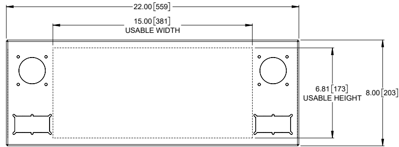
P/N: FMP-22-A-UNCUT
