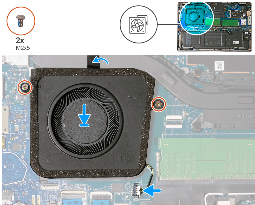
Figur 25. Installera fläkten
