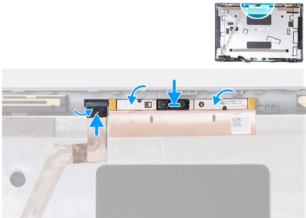
Figur 59. Installera kameramodulen
