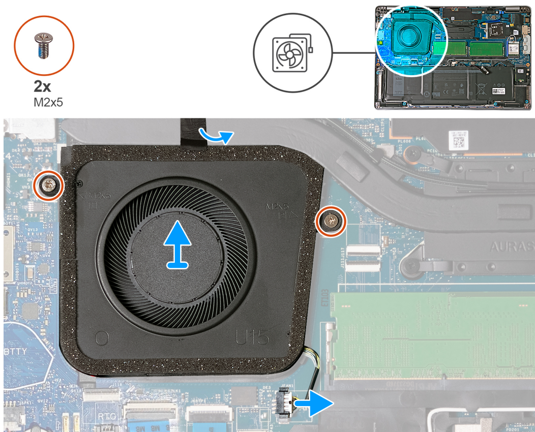
Figur 24. Ta bort fläkten
