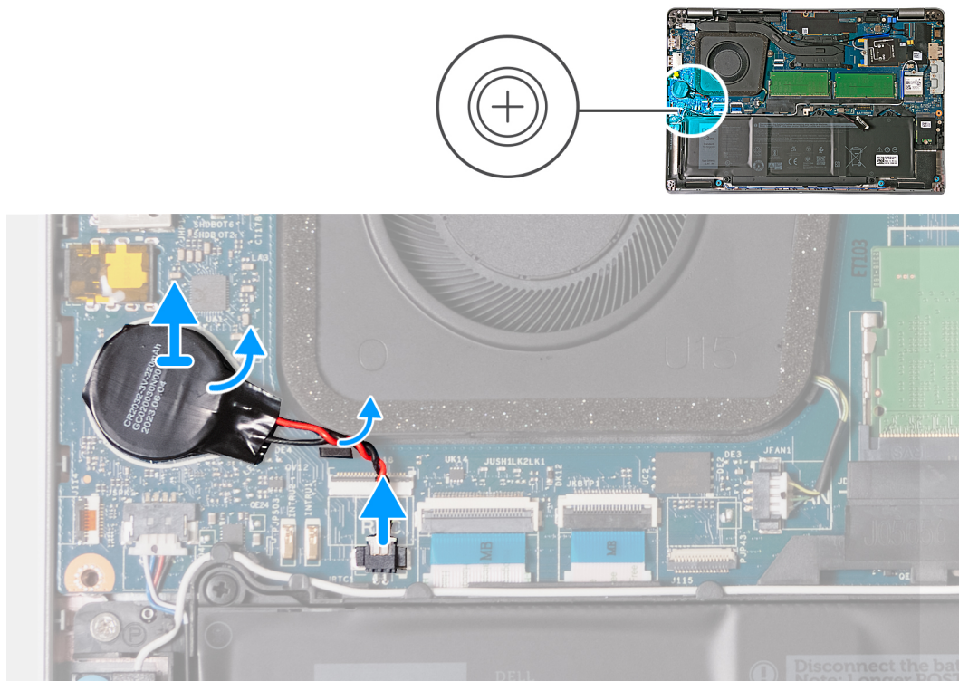
Figur 28. Ta bort knappcells batteriet
