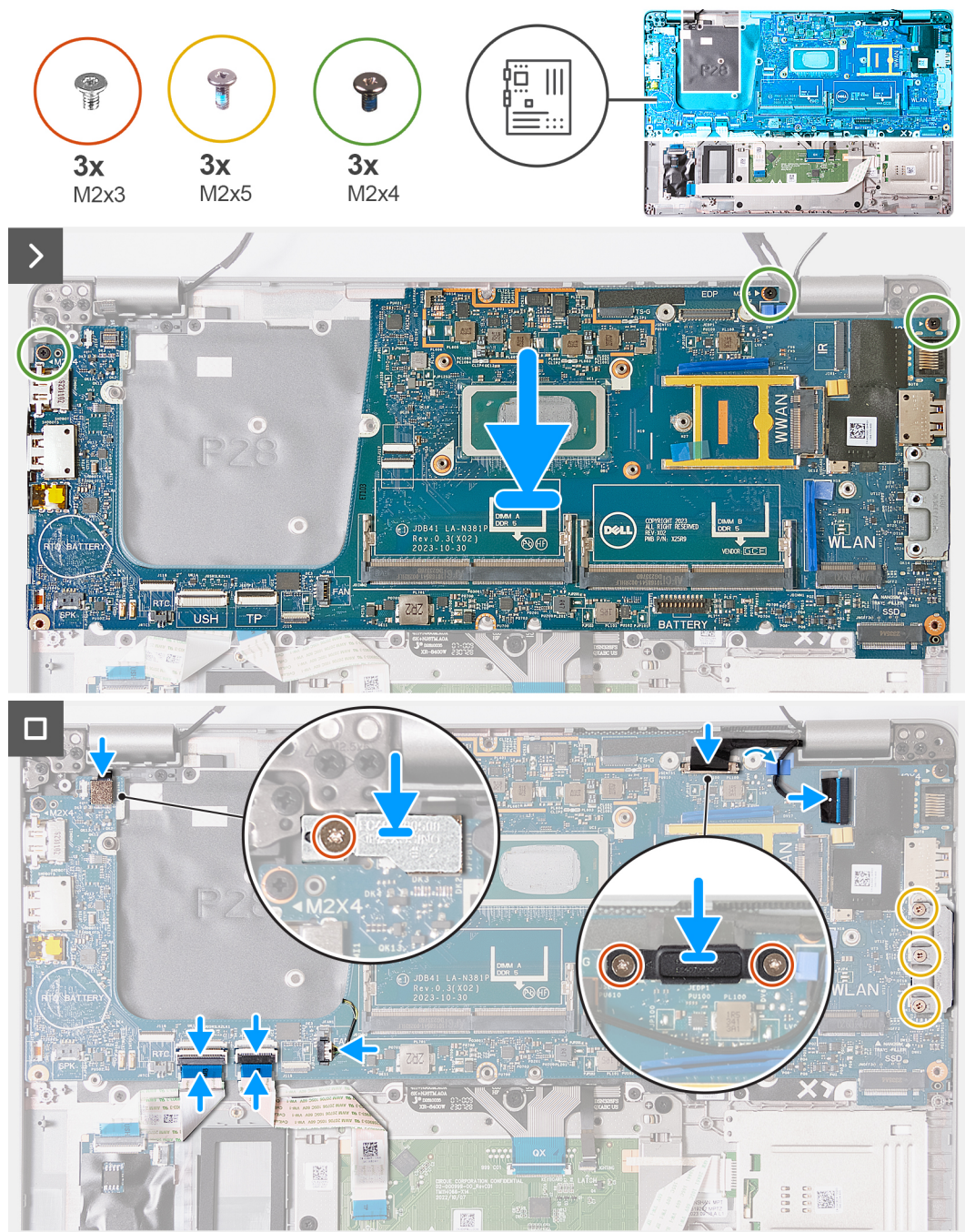
Figur 72. Installera moderkortet
