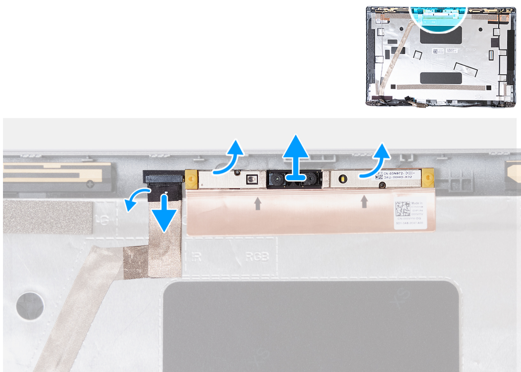
Figur 58. Ta bort kameramodulen
