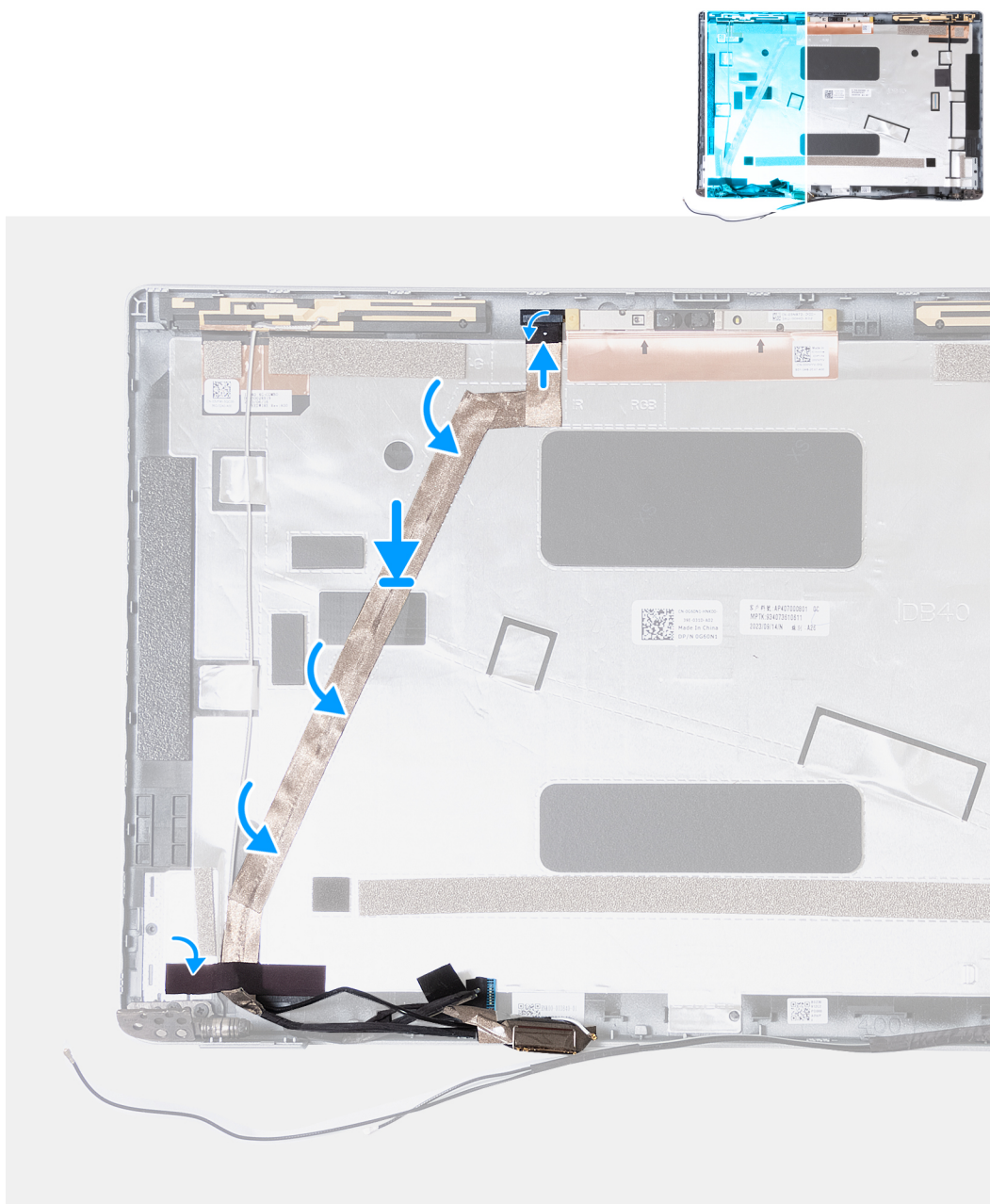
Figur 63. Installera bildskärmskabeln
