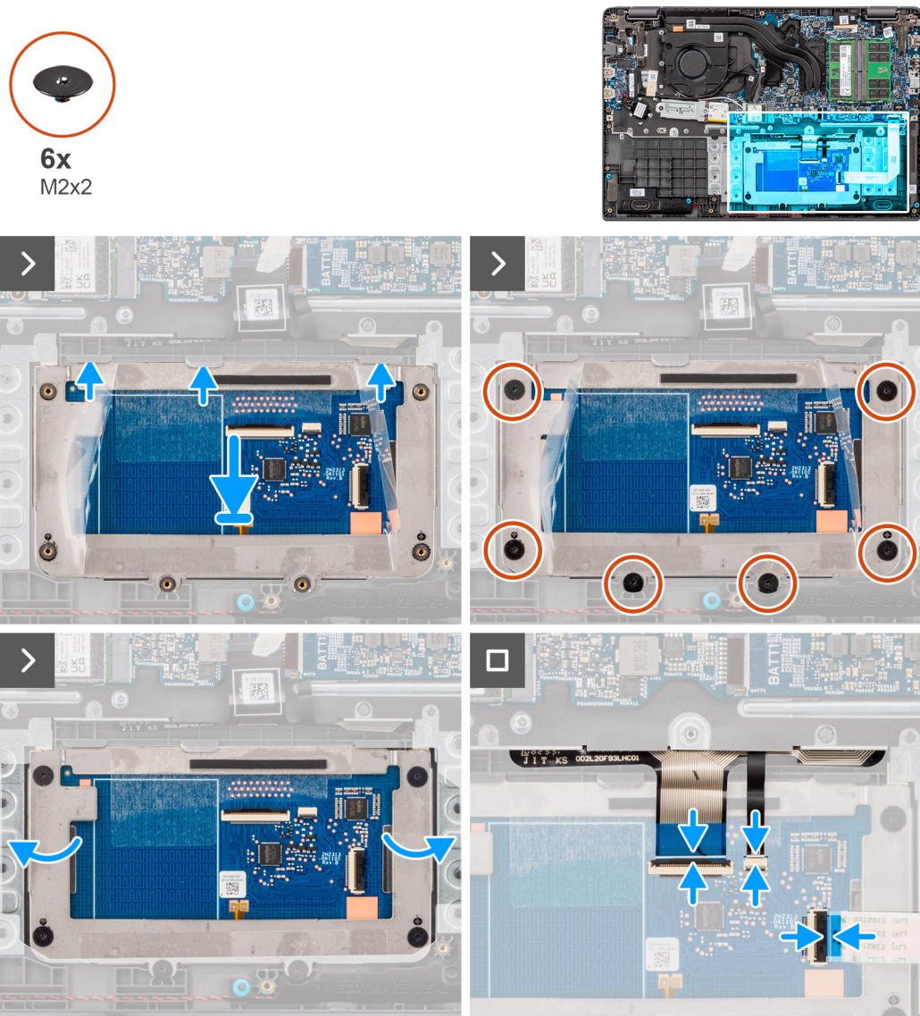
Figur 36. Installera styrplattan
