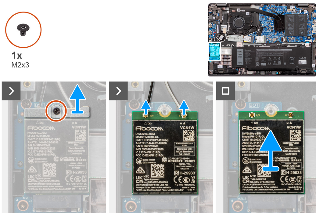
Figur 16. Ta bort WWAN-kortet
