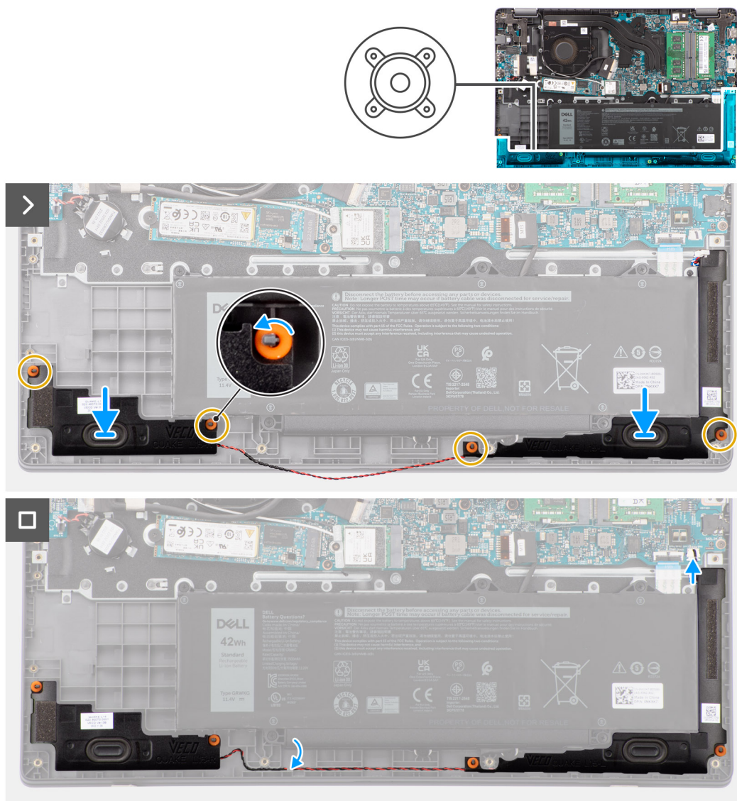
Figur 21. Installera högtalarna
