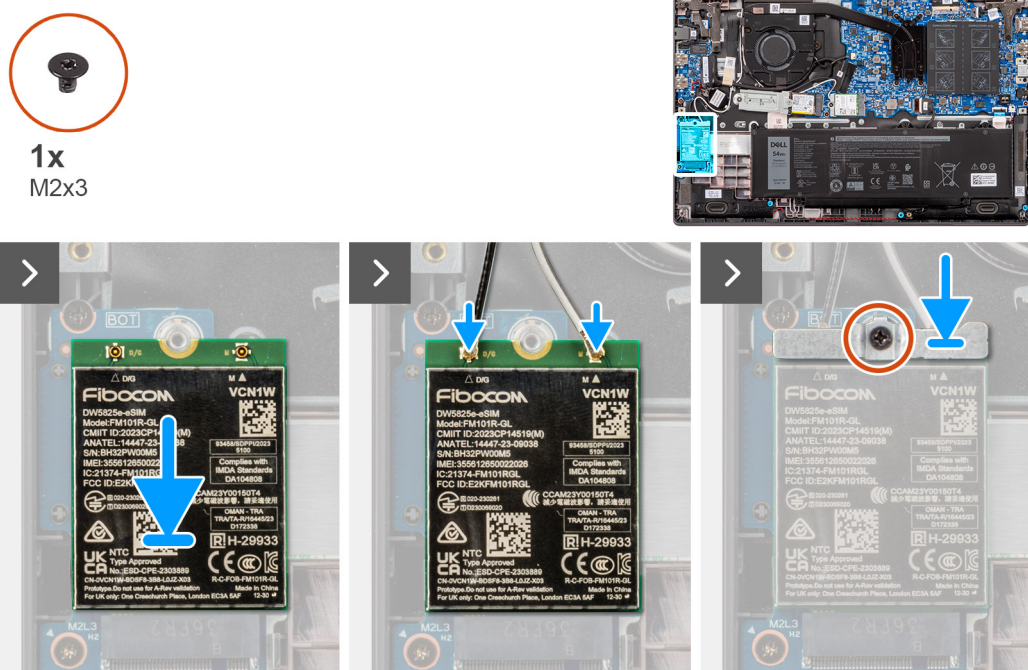
Figur 17. Installera WWAN-kortet
