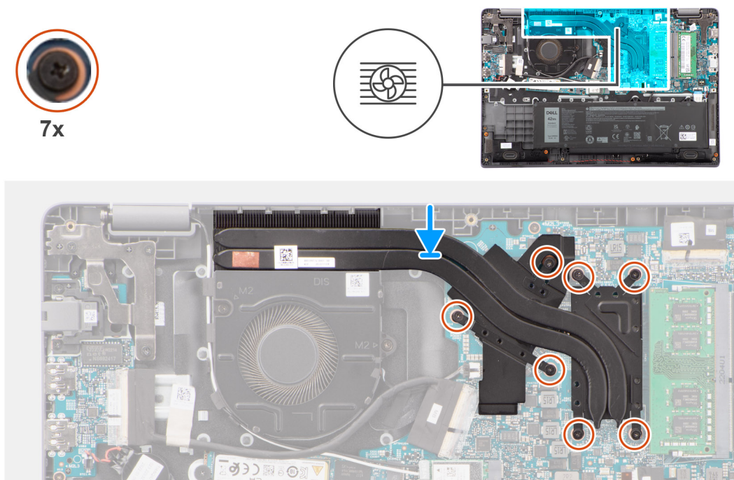
Figur 32. Installera kylflänsen för diskret grafikkort
