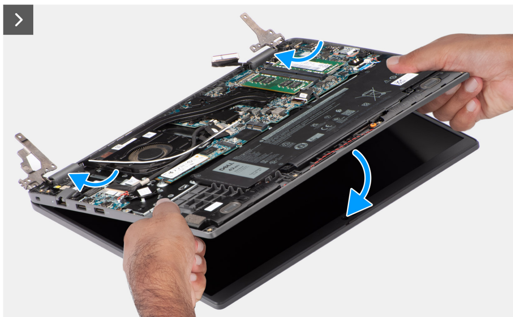
Figur 51. Installera bildskärmsenheten
